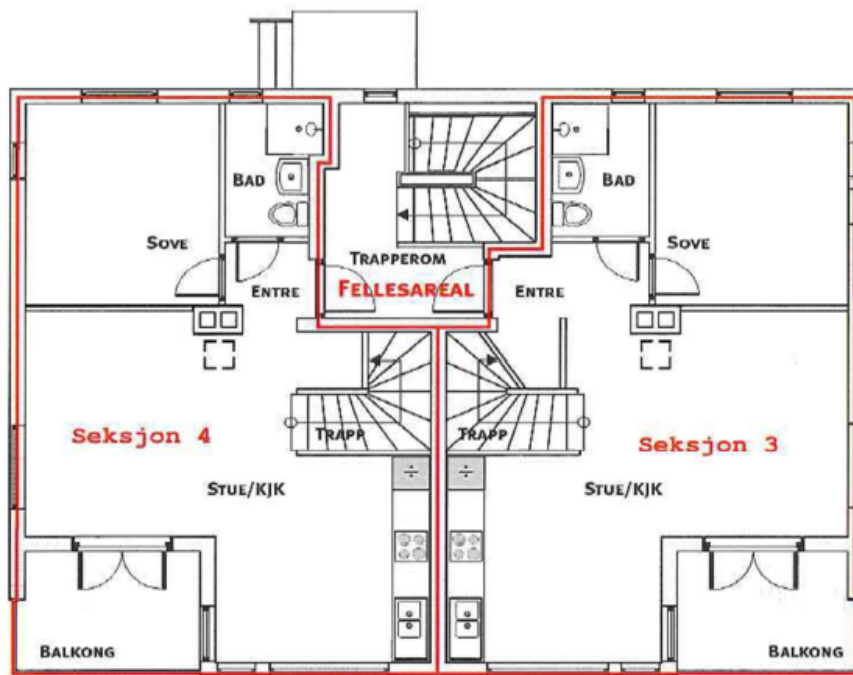
2. Etasje
