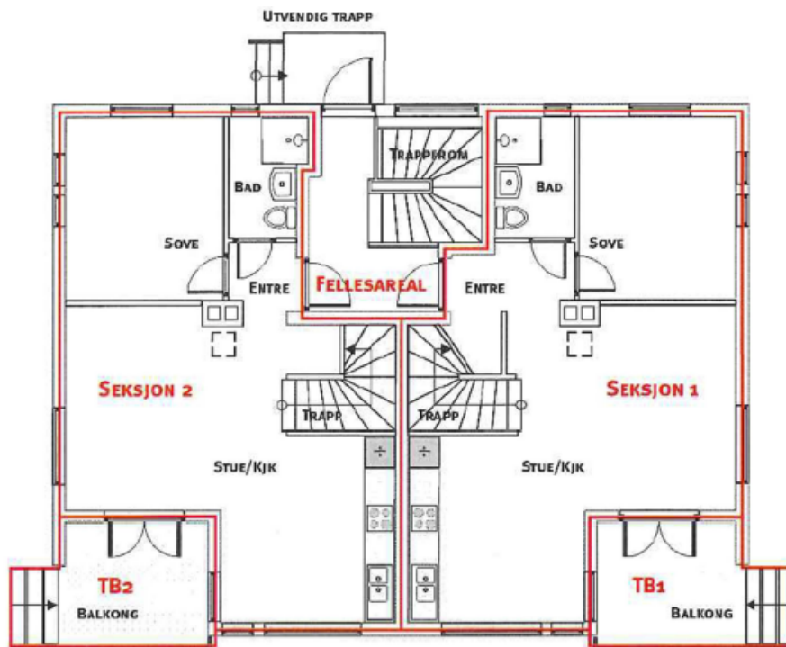
1. Etasje
