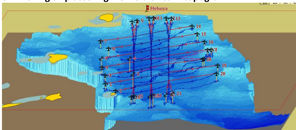
Tredimensjonal bunntopografi med fortøyninger ved Helsøya II sett fra nordøst. Kartkilde: Olex
